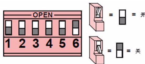
图 4.1 DX3010-CHI 地址设置
