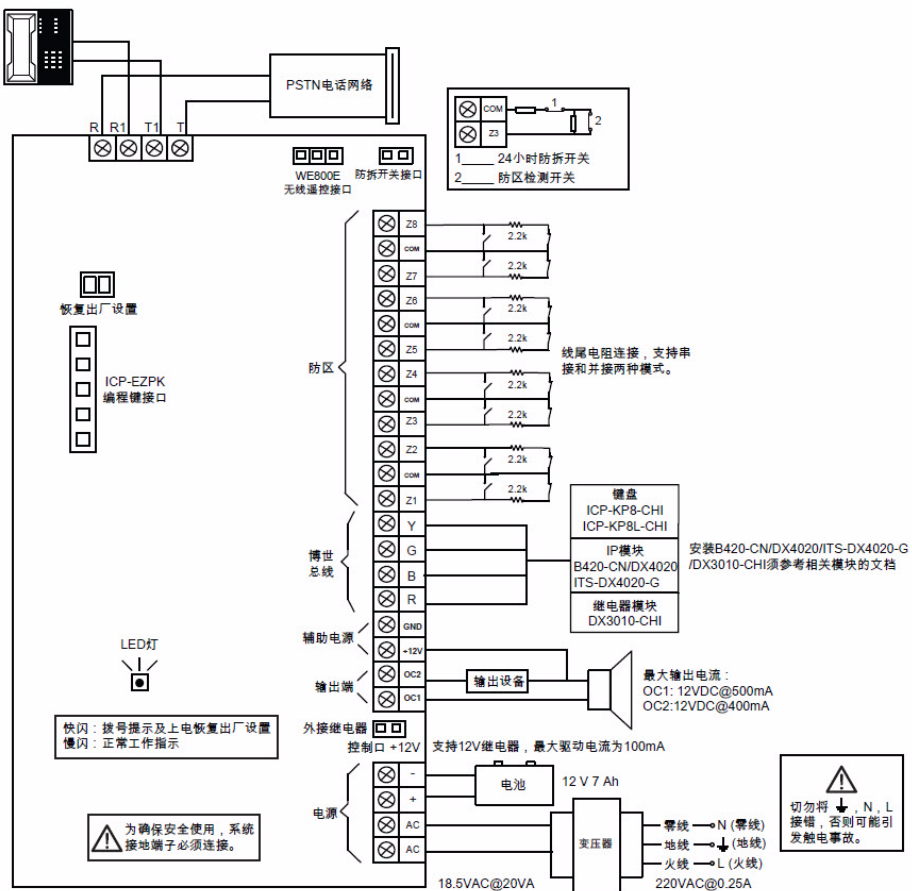
图 18.1 接线图
