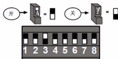
图 4.2 DX4020 地址设置
